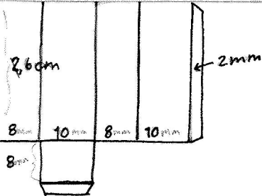
laatikon runko LÄDÄNS YTERHÖLJE
